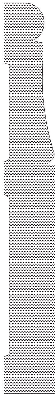
BLBB035 7/8" x 7"
