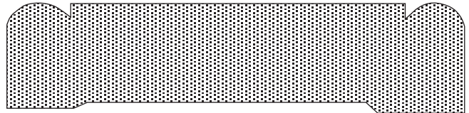
BLCS089 11/16" x 3-5/16"
